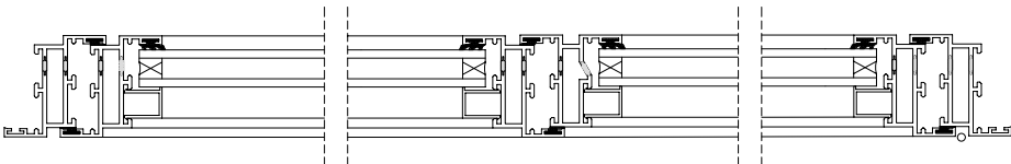
D.1 DETALLE DE CARPINTERIA 1/5
