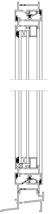
D.2 DETALLE DE CARPINTERIA 1/5
