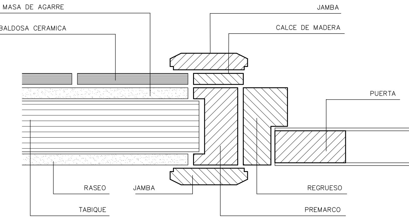
DETALLE.- ESCALA 1/2 (PARA LOS CASOS DE BAÑOS Y COCINAS DONDE VAYA COLOCADA BALDOSA CERAMICA)
