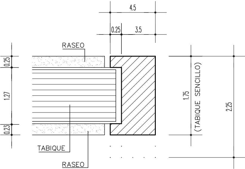
PREMARCO ESCALA 1/2
